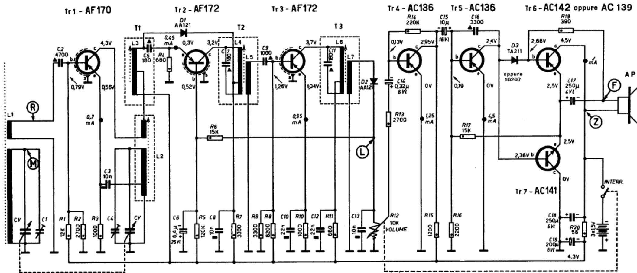
Schema elettrico del radiorecettore PHONOLA mod. RT1760 Poker
